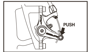
D-3 Check arm return
